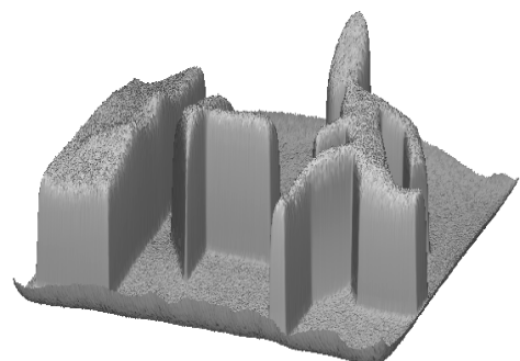
Bild 3: Leuchtdichteverteilung
