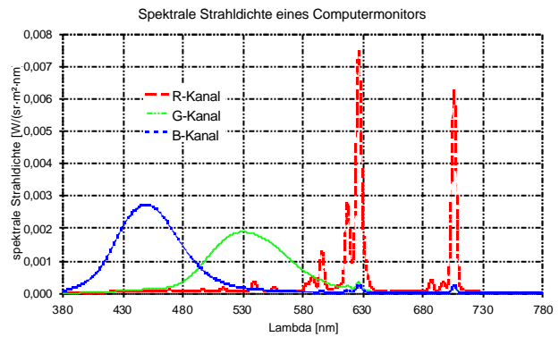
Abb. 9: Spektrale Strahlidichte eines CRT-Monitors
