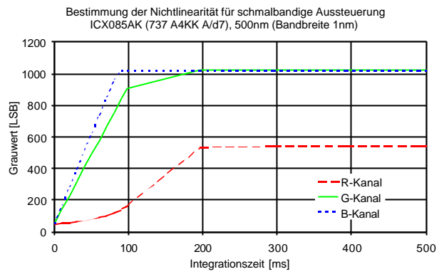
Abb. 12: Bestimmung der Nichtlinearität für schmalbandige spektrale Strahldichten
