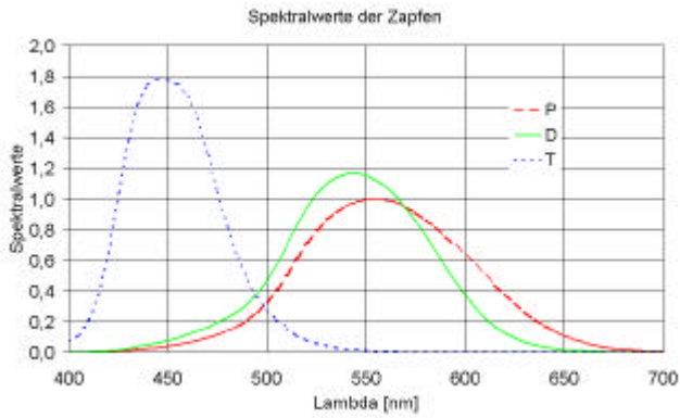
Abb. 3: Augenempfindlichkeit des 2°-Normalbe- trachters
