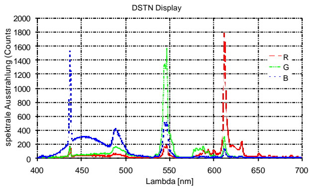
Abb. 8: Spektrale Strahlidichte eines DSTN-Displays
