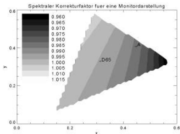
Abb. 1: Notwendiger Korrekturfaktor, durch die spektrale Ausstrahlung bei Monitormessungen
