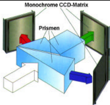
Abb. 5: Strahlteilerwürfel einer 3Chip CCD-Kamera
