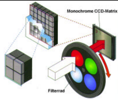
Abb. 7: Anwendung eines Filterrades /AGFA/
