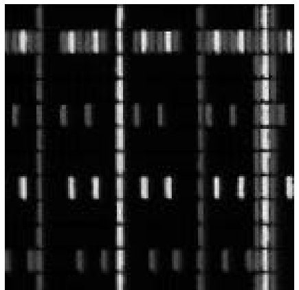
Abb. 15: Mikrostruktur eines TFT-Displays (links linear skaliert, Mitte log. Skaliert über 4 Dekaden, rechts Luminanz (linear))
