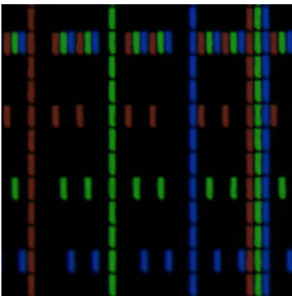
Abb. 15: Mikrostruktur eines TFT-Displays (links linear skaliert, Mitte log. Skaliert über 4 Dekaden, rechts Luminanz (linear))
