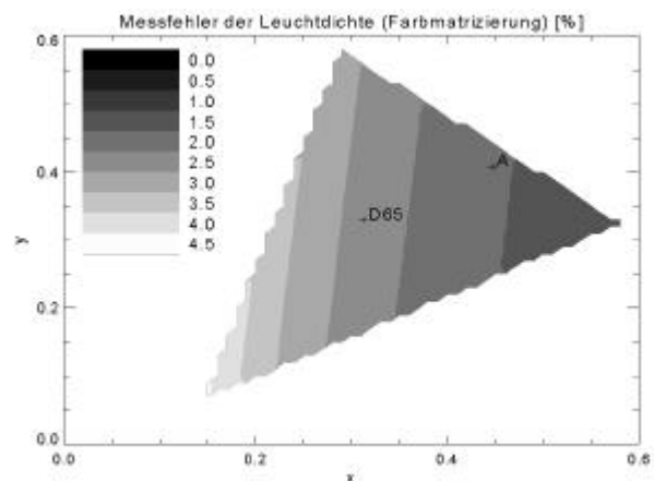
Abb. 2: Meßfehler, durch die spektrale Bewertung bei optimaler Matrizierung
