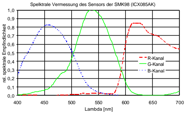
Abb. 11: Relative spektrale Empfindlichkeit der einzelnen Pixelklassen (ICX085AK)
